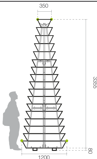
A Seitenansicht
