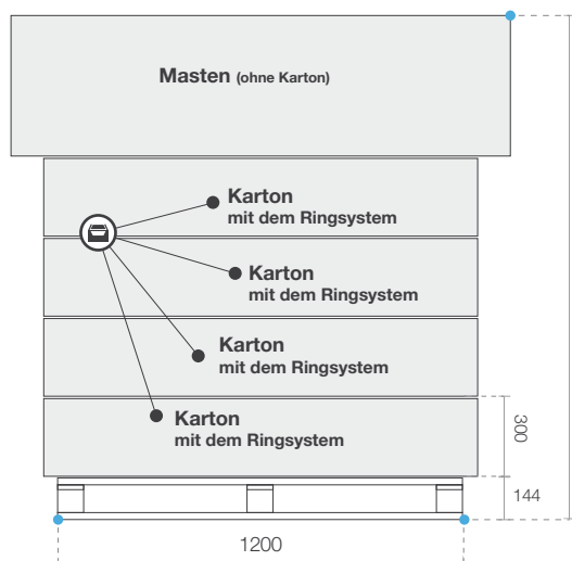
A Seitenansicht
